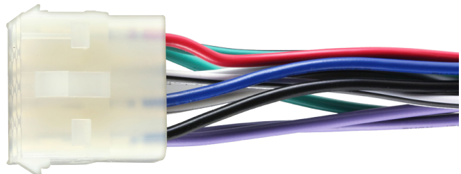
Plug/Wire Bundle vue de côté (photo)
